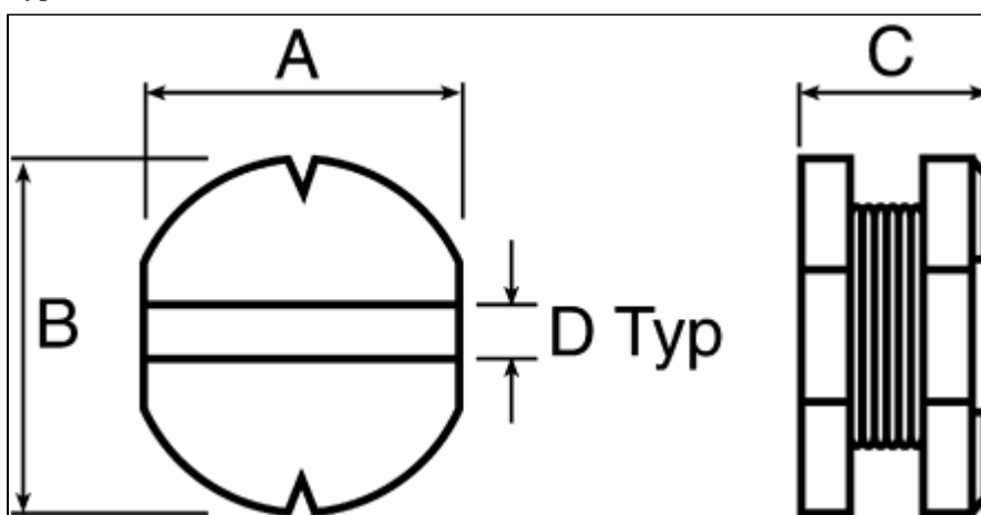
Typ XL (offene Bauform)
