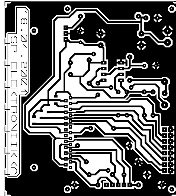
PIIRILEVYN FOLIOKUVA JUOTOS- PUOLELTA KATSOTTUNA.
