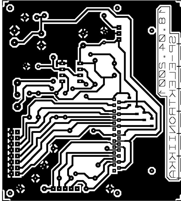
PIIRILEVYN FOLIOKUVA KOMPONENTTI- PUOLELTA KATSOTTUNA.
