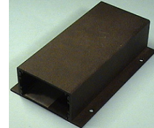
Alumiinikotelo, pulverimaalattu musta, kaksi korttiuraa sisällä, kiinnitys reunukset, ei päätylevyjä, erittäin hyvä kotelo suodattimille, vahvistimille, RF -käyttöön ym. mitat, (ei sisällä kiinnitys reunusten leveyttä.) kork. 33, lev. 54.5, syv. 120 mm. (SRF3) 4.50€
