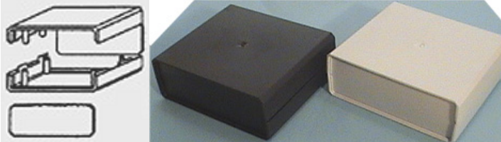
Muovikotelo (37), "MITTALAITEKOTELO", muovi tassut, irrotettavat etu- ja takalevyt, ulkomitat n.60x160x140 mm, materiaalipaksuus n.3mm. Musta (37): 4.50€ Vaalea (37A): 6.80€
