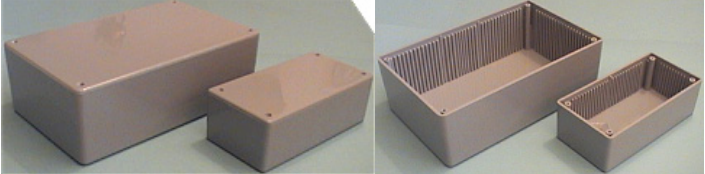
Siniharmaat muovikotelot, korttiurilla, 45 x 65 x 130 mm, yleiskäyttöinen muovikotelo pienilaitteille. Muovikotelo (33) 3.50€ Muovikotelo siniharmaa, 65 x 115 x 185 mm. Muovikotelo (34) 6.50€
