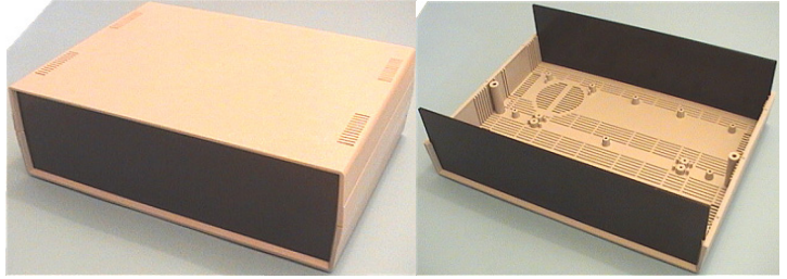
Muovikotelo (40), "MITTALAITE / VERKKOLAITE" kotelo, vaalean sävyinen tyylikäs, mustat etu ja takalevyt, jäähdytysaukot, kaiutin/tuuletin ritiläaukko, sisällä kiinnityspaikkoja ja uria piirilevyille. lev.255 mm x syv.190 mm x kork.83mm. Mittapiirustukset nettisivuillamme . Muovikotelo (40) 10.90€
