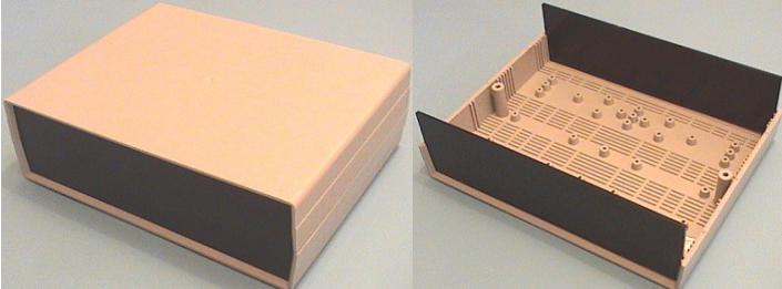
Muovikotelo (39), "MITTALAITE / VERKKOLAITE" kotelo, vaalean sävyinen tyylikäs, mustat etu ja takalevyt, kaiutin/tuuletin ritiläaukko, sisällä kiinnityspaikkoja ja uria piirilevyille, lev.200 mm x syv.160 mm x kork.65 mm. Mittapiirustukset nettisivuillamme . Muovikotelo (39) 8.40€
