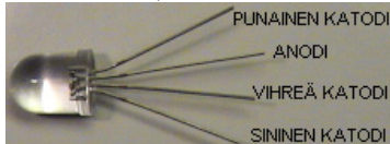
RGB-LED:in jalkajärjestys
